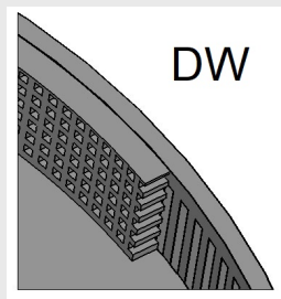
Doppelwand Double paroi Double outer wall
